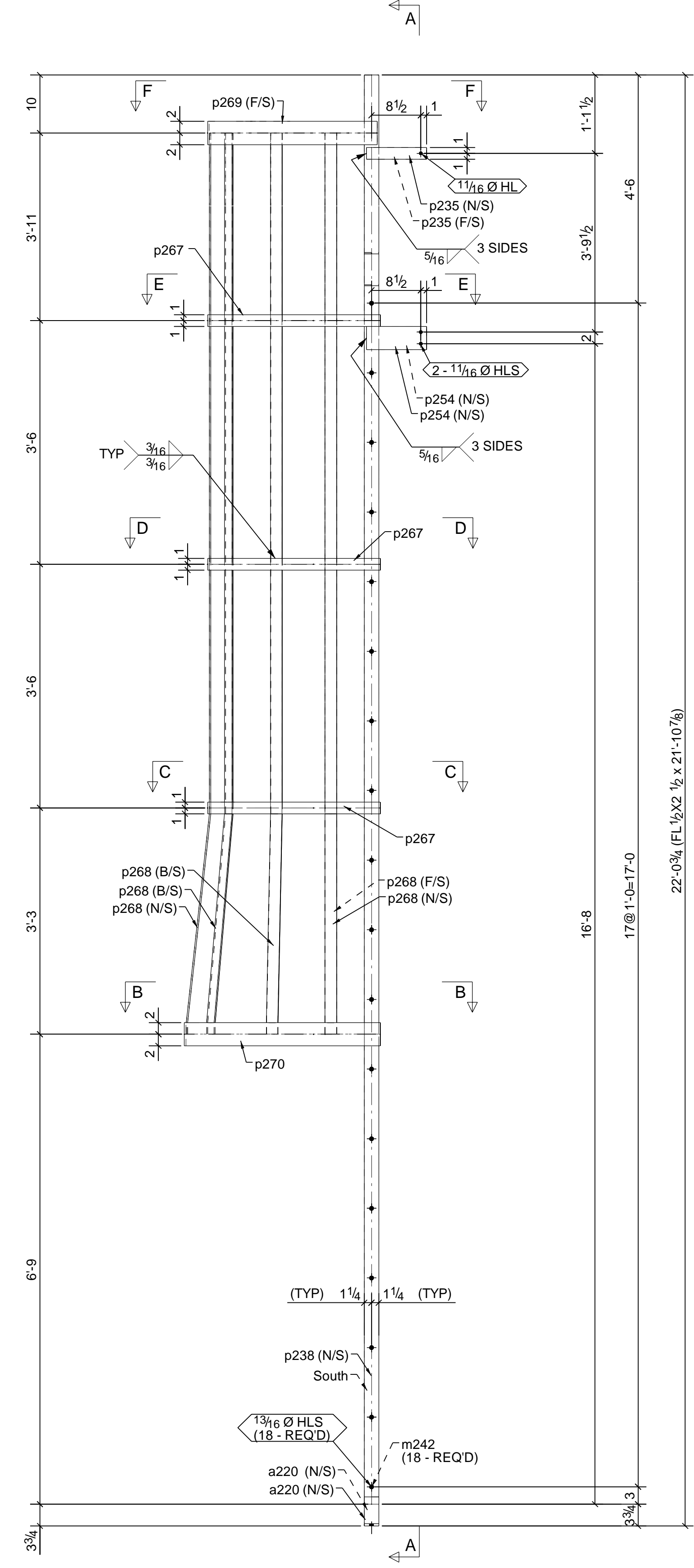
ONE - LADDER - 437LD1
