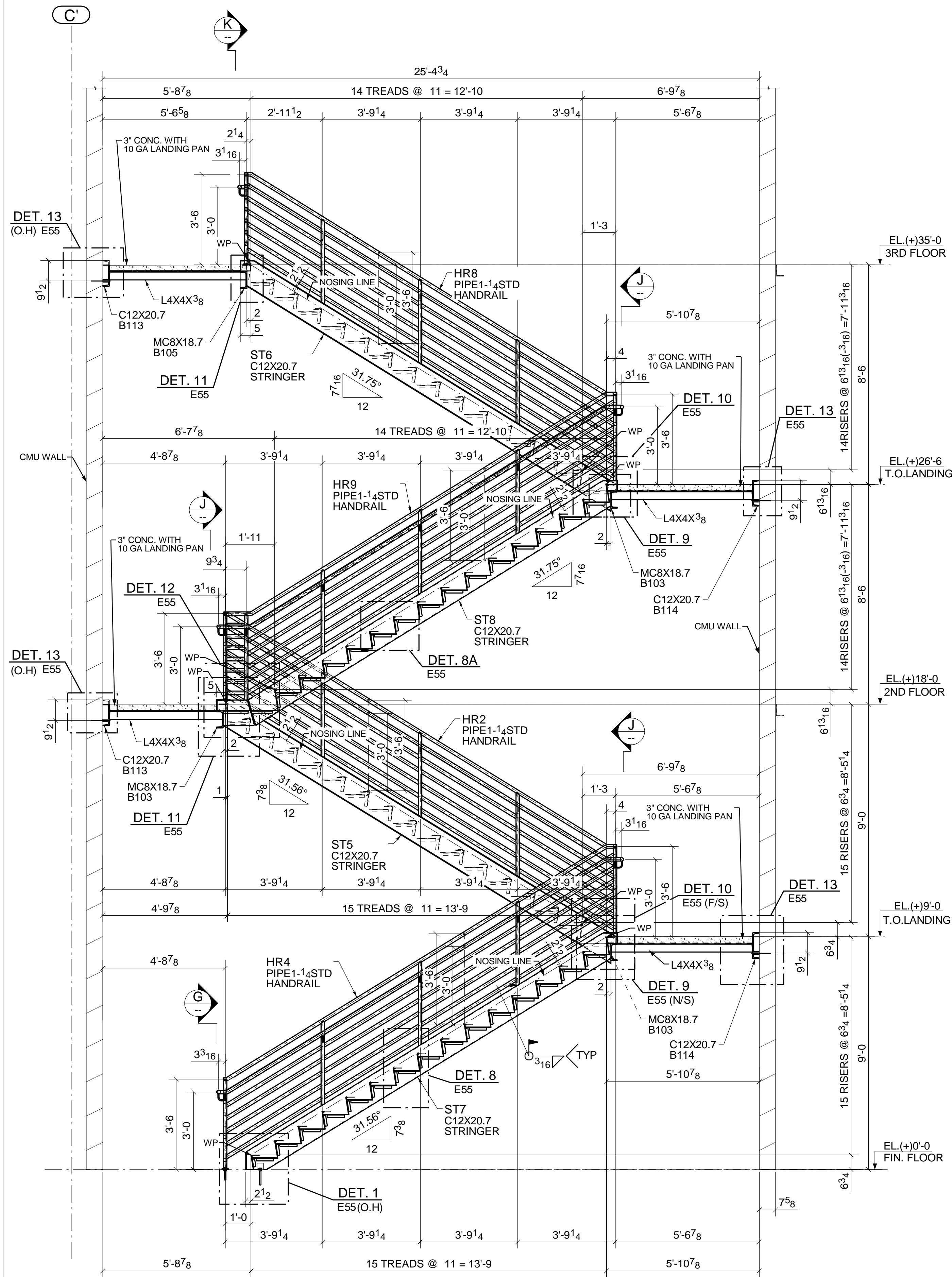
SECTION C - C (REF: E51 & E52)
